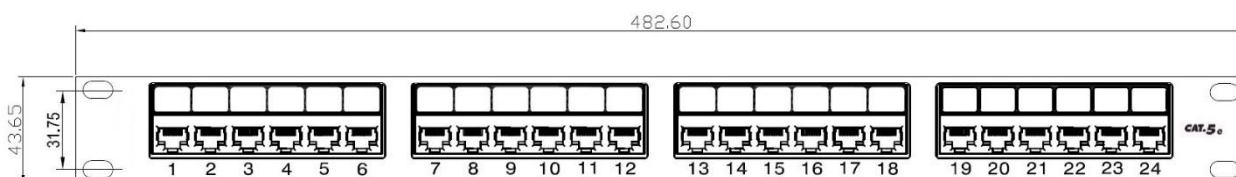
Рисунок 2. Монтажно-габаритные размеры коммутационной панели 24458ЕС-С5Е
