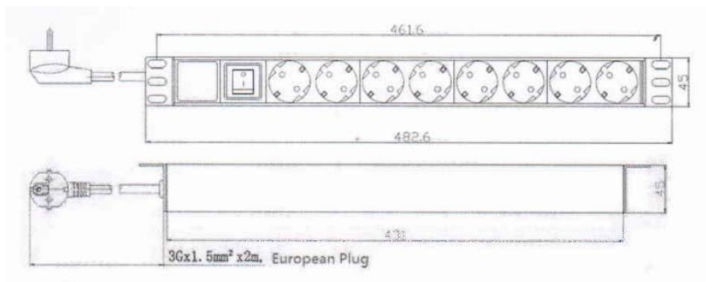
Рисунок 2. Монтажно-габаритные размеры блока розеток REC-S816
