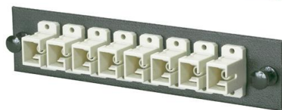
Рис.2: Вставки монтажные под ST и SC разъемы
